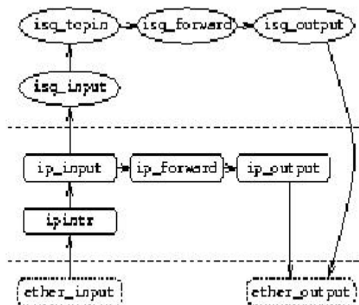
Gambar 2: Aliran data melalui FreeBSD kernel yang dimodifikasi
